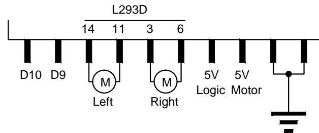
Schema connettore
